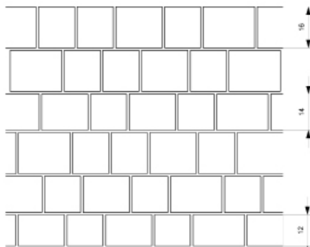
Détail du pavage en calcaire marbrier
