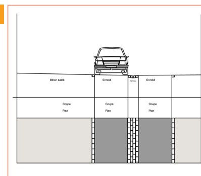
Profil des voies routières
