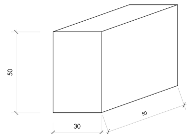
Détail des bornes en pierre calcaire de pays
